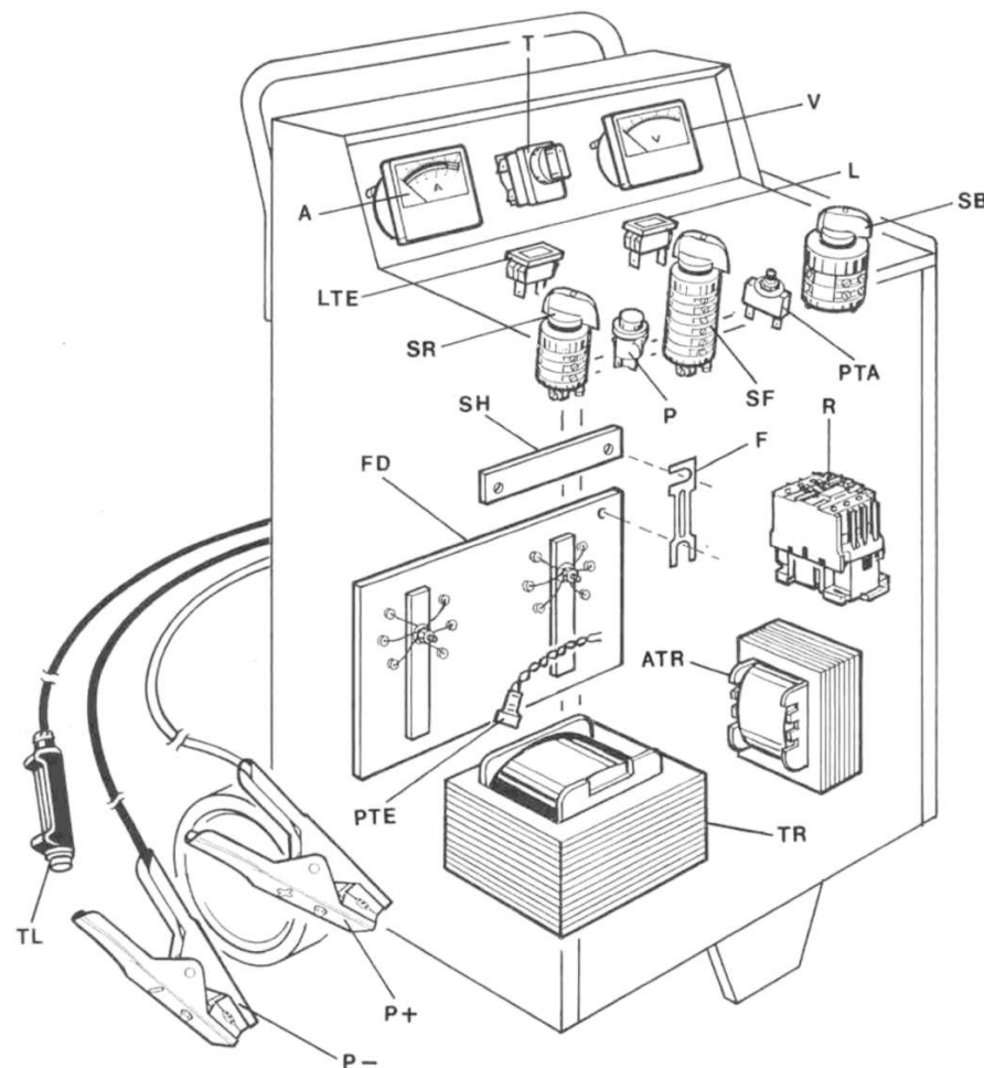
Elenco ricambi mod. START 500
